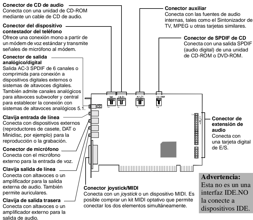
Clavijas y conectores de la tarjeta SB Live! Player 5.1.
