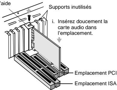
Fixation de la carte son dans l'emplacement d'extension PCI.
