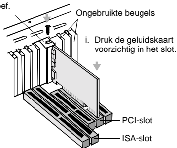
De audiokaart vastzetten in de PCI uitbreidingsleuf.
