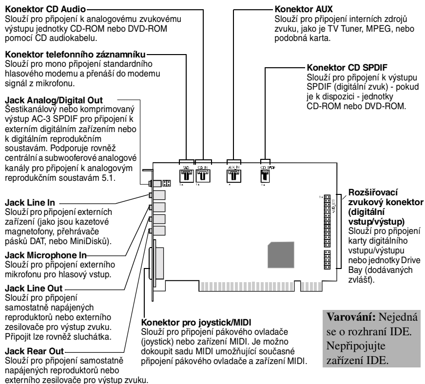
Jacky a konektory na kartě SB Live! Player 5.1.
