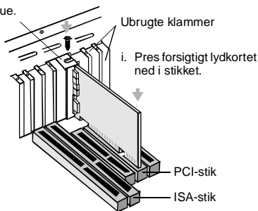
Fastgørelse af lydkortet til PCI-udvidelseskortpladsen.
