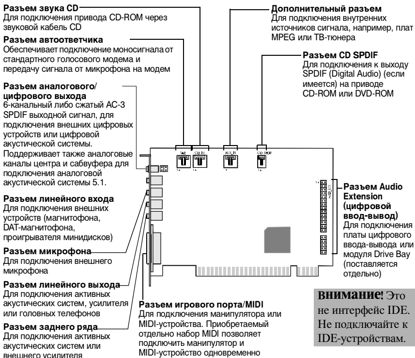
Расположение гнезд и разъемов на звуковой плате.
