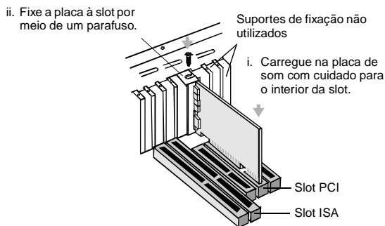
Fixação da placa de som na ranhura de expansão PCI.
