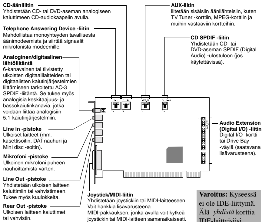
SB Live! Player 5.1 -äänikortin liittimet
